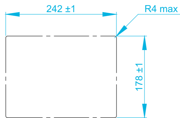
Einbau-Ausschnitt OPC8008 Mounting-Cutout OPC8008
