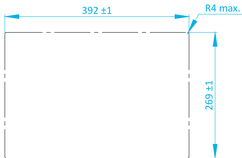
Einbau-Ausschnitt OPC8015 Mounting-Cutout OPC8015
