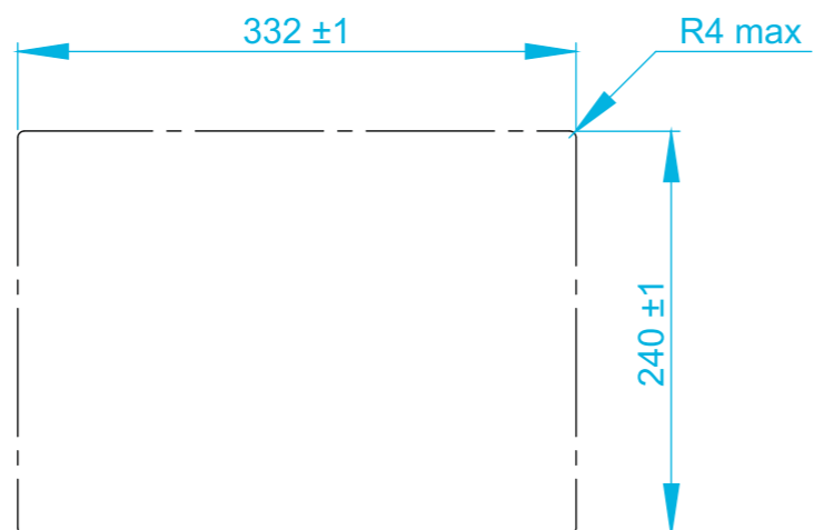
Einbau-Ausschnitt OPC8013 Mounting-Cutout OPC8013
