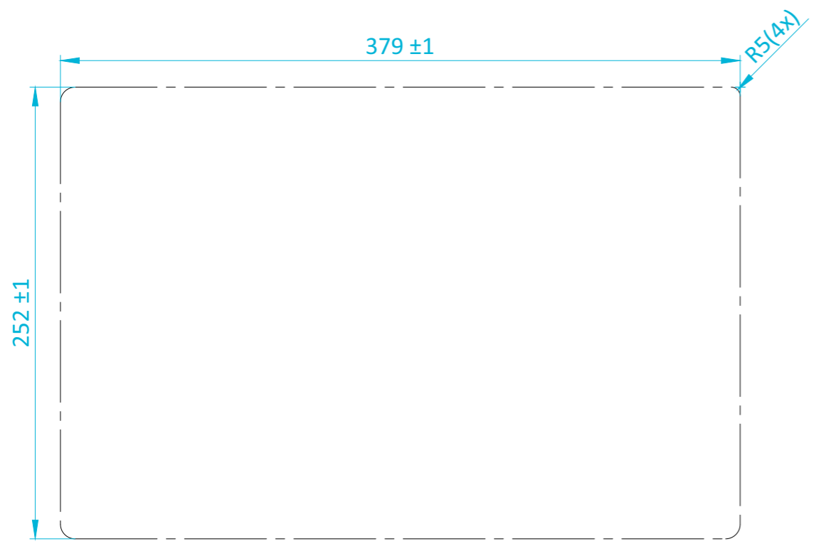
Einbau-Ausschnitt OPD9016 Mounting-Cutout OPD9016
