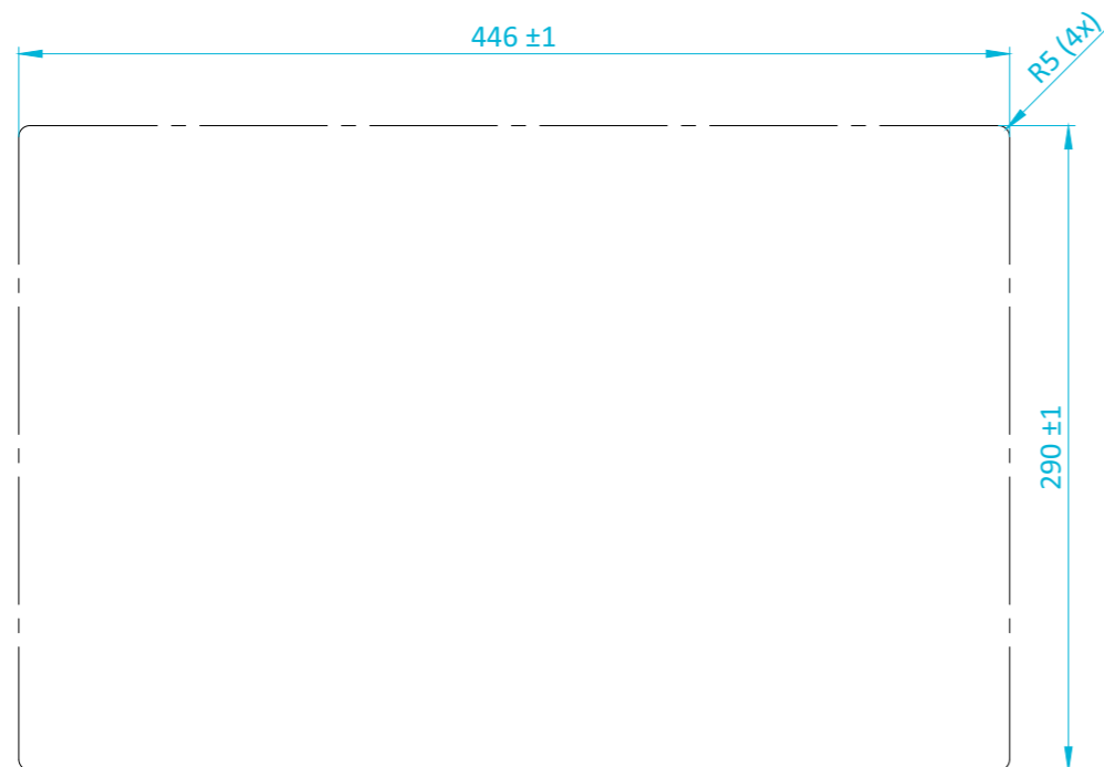
Einbau-Ausschnitt OPD9019 Mounting-Cutout OPD9019
